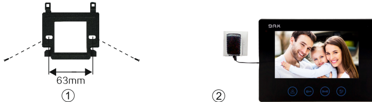
rys. 3 Montaż monitora
