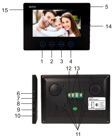
rys. 1 Budowa wideo monitora
