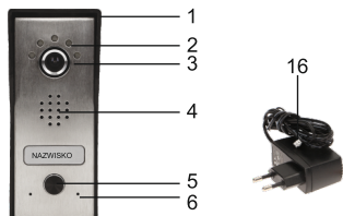
rys. 2 Budowa panelu zewnętrznego
