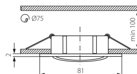
NAVI CTX-DT10-C/M
