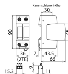
Rysunek wymiarowy DG M H TT 2P 275 FM
