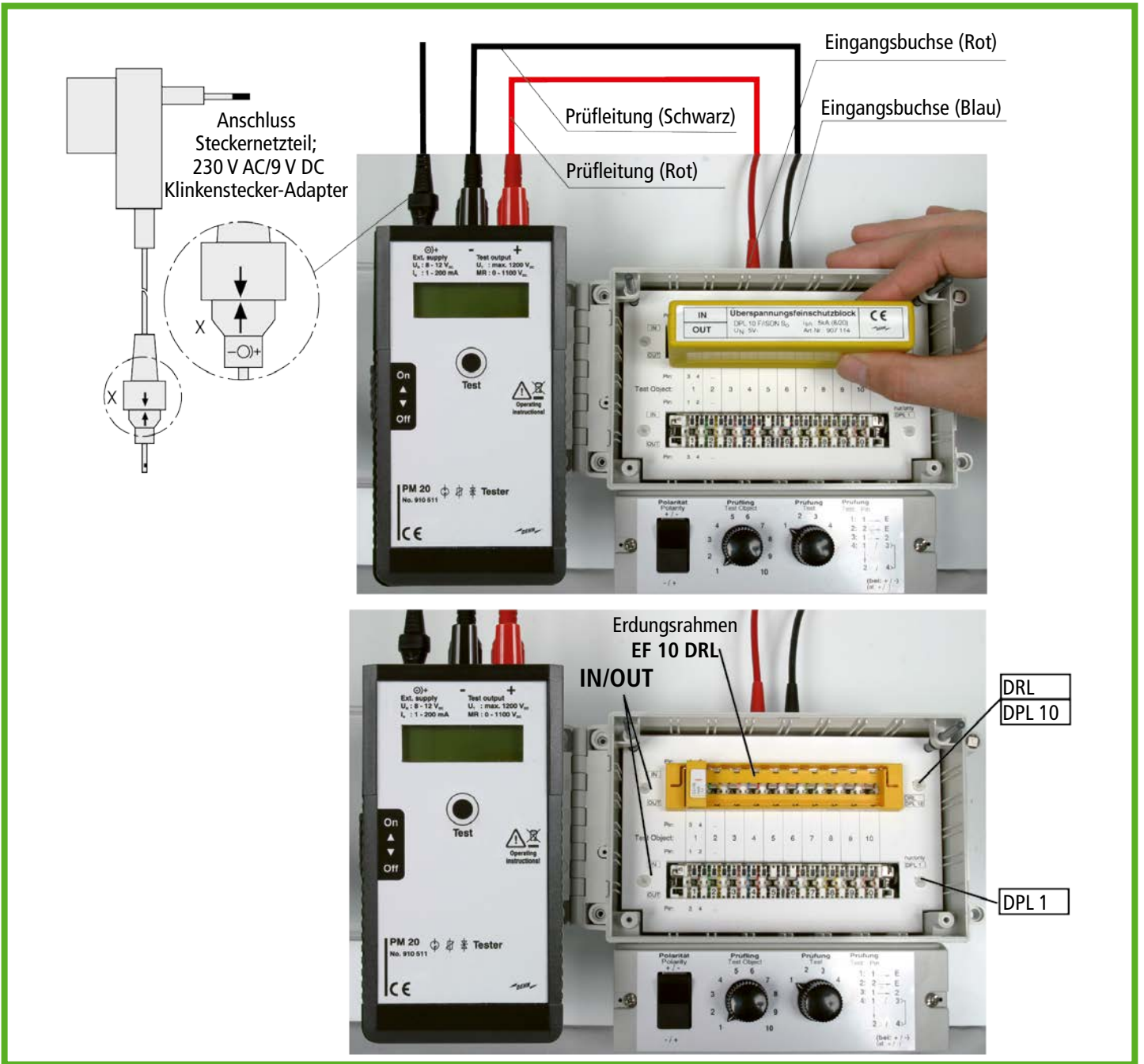
Figur 4 Prüfaufbau 2
