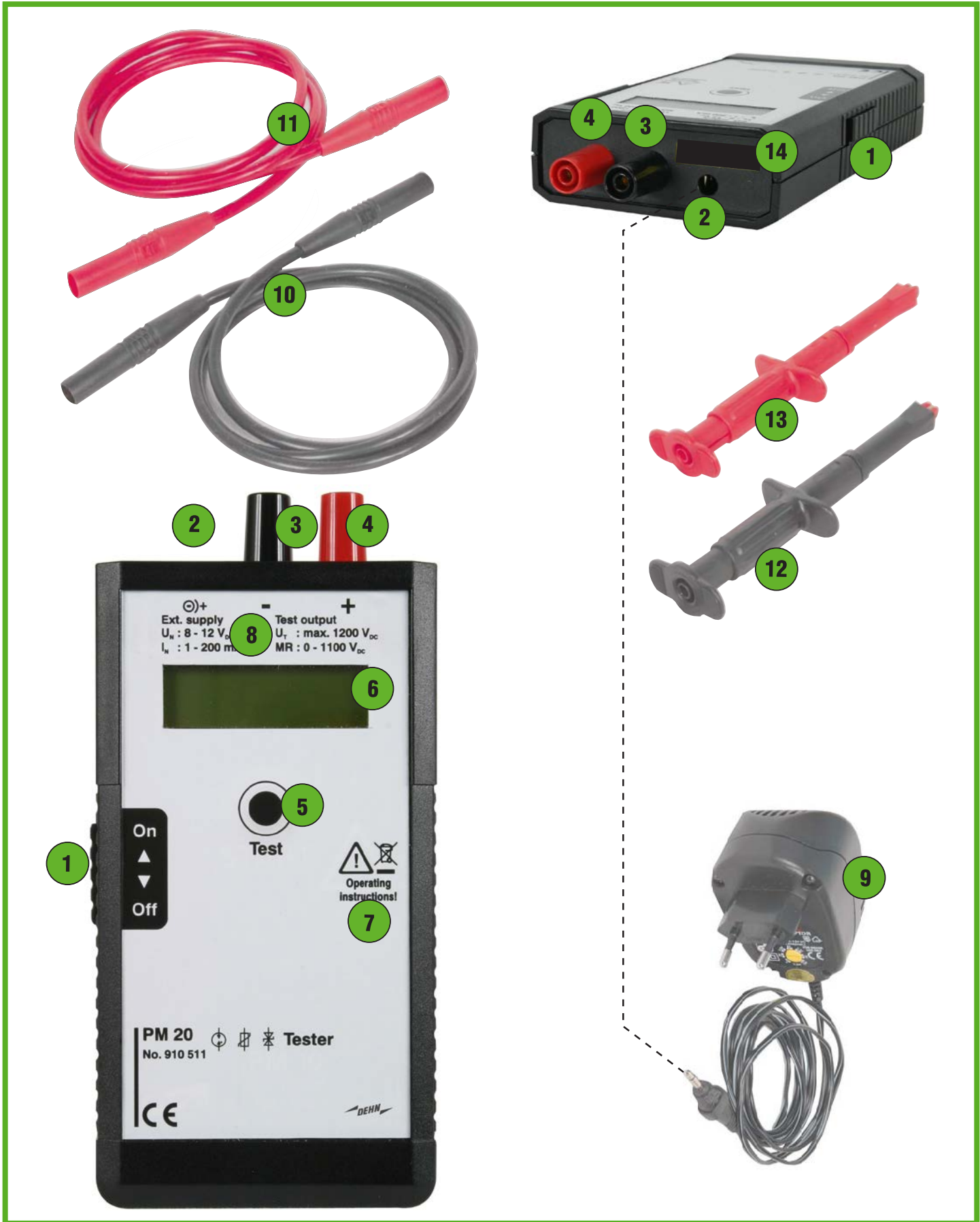
Figur 2 Gerätebeschreibung
