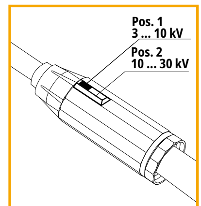
Bild 10 Nennspannungswahlschalter
