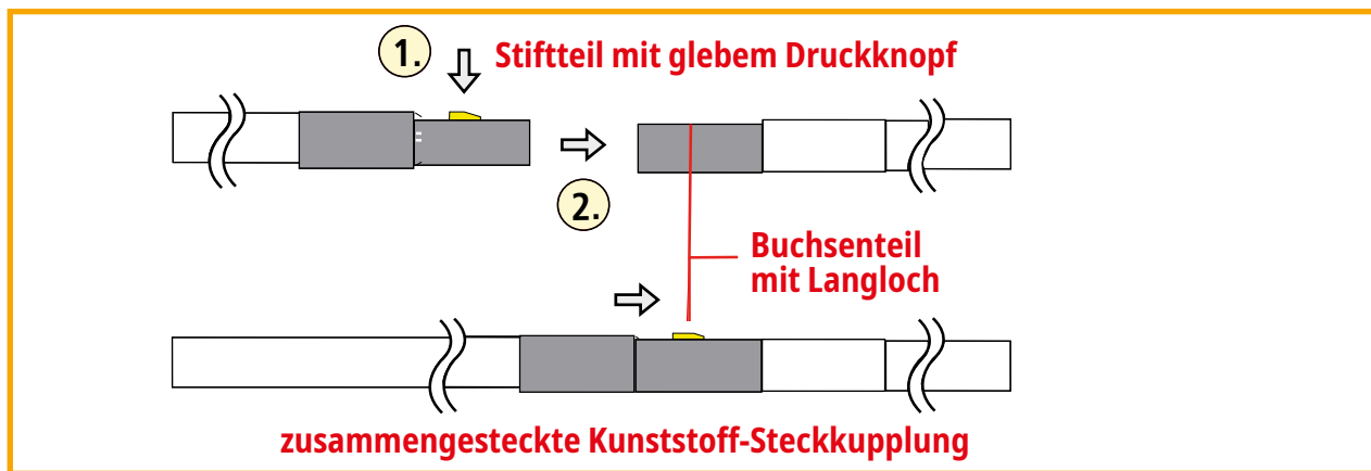
Bild 7 Steckkupplungs-System
