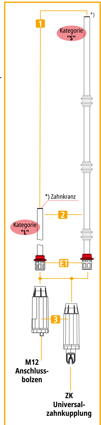
Bild 4 Aufbau
