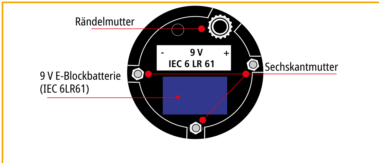
Bild 13 Unterseite Elektronikteil
