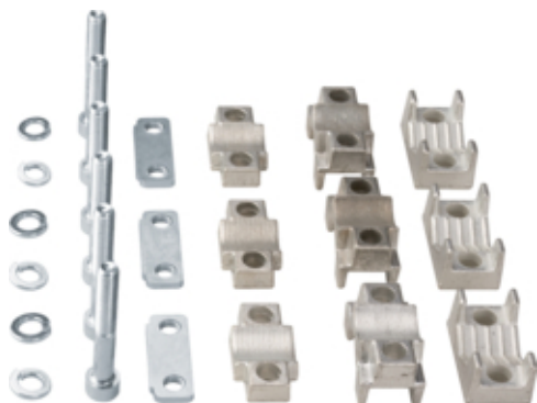
LT zestaw zacisków pryzm. do rozłącz. NH2 (3 szt.) 2x70-120mm 2 Cu/Al 2 przewody
