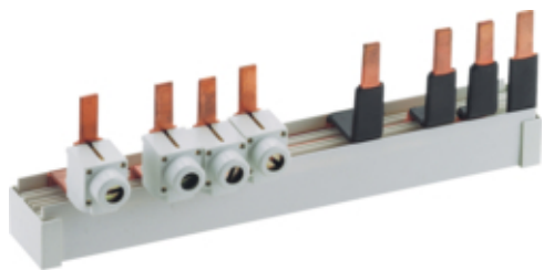
Szyna sprzęgająca
