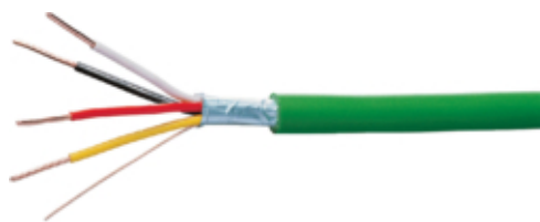
KNX e/s Kabel magistralny KNX-BUS, 500 m
