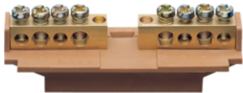
Zaciski fazowe 4x16+4x10
