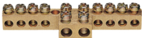
Listwa przyłączeniowa bez wspornika 2x2x16 + 8x10 mm 2
