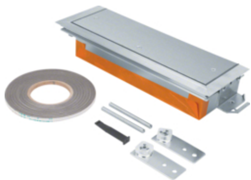
tehalit.BK Końcówka kanału wanna stalowa BKWD 300x(80-120)mm stal
