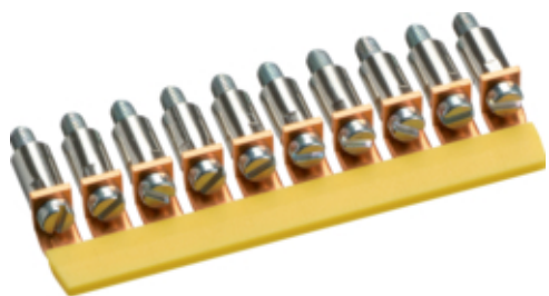
Mostek równoległy 10-polowy do zacisków 4mm 2
