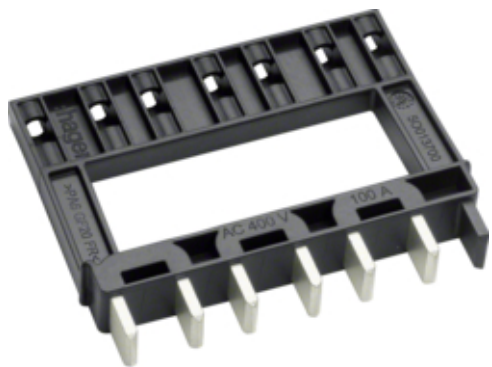
Mostek zwierający do listwy KJ30x (3+N)
