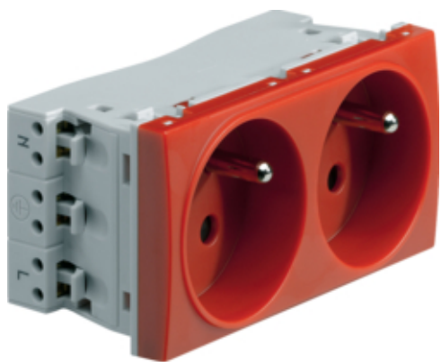
systo Gniazdo przelotowe z uziemieniem 2x(2P+Z) 16A/250V samozaciski 4M czerwony
