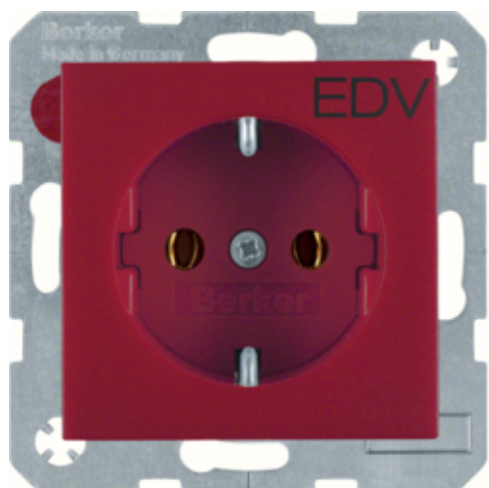
S.1/B.3/B.7 Gniazdo SCHUKO z nadrukiem 'EDV', czerwony
