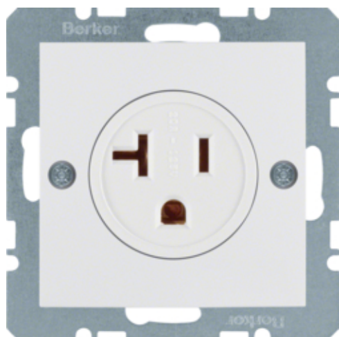
B.Kwadrat/S.1 Gniazdo z uz. USA/KANADA NEMA 5-20 R, biały
