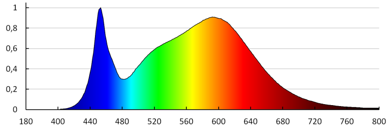
KANLUX S.A. (kat 33753) DULI LED 6,5W-NW-O-GR / LDC (Polar)
