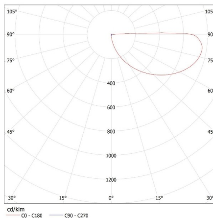
KANLUX S.A. (kat 33753) DULI LED 6,5W-NW-O-GR / LDC (Polar)
