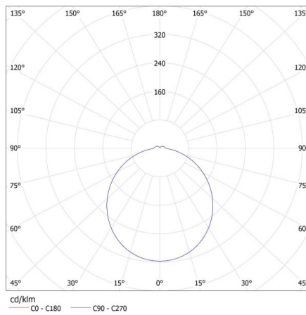
KANLUX S.A. (kat 26440) VARSO LED 18W-WW-O / Krzywa rozsytu światła (biegunowo)
