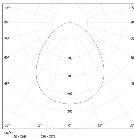
KANLUX S.A. (kat 25782) IVIAN LED 4,5W W-NW / LDC (Polar)
