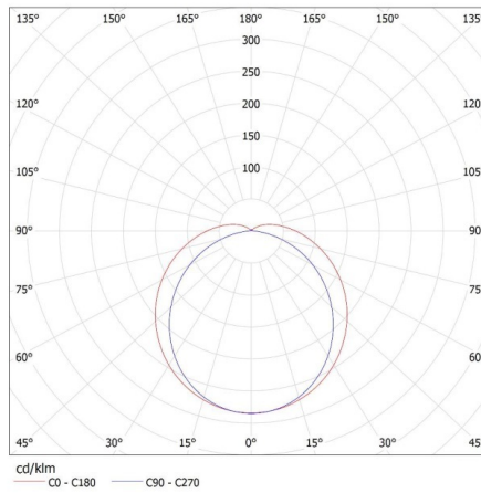
KANLUX S.A. (kat 22604) MAH-LED N 40W-NW / Krzywa rozsytu światła (biegunowo)
