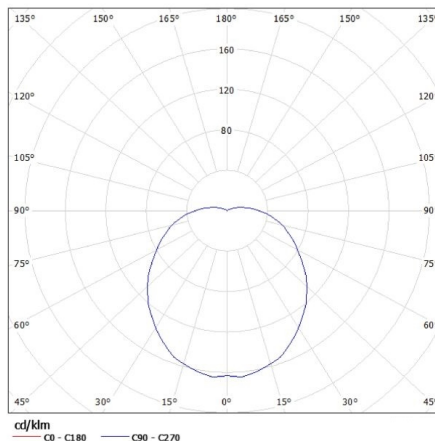
KANLUX S.A. (kat 18120) FOGLER DL-2400 / Krzywa rozsytu światła (biegunowo)
