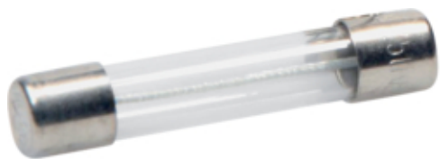
Wkładka bezpiecznikowa szklana F wyk.szybkie 6,3x32mm 0,1A 250 VAC/DC
