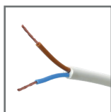
przewód o izolacji polwinitowej (H05VV-F) 2x1.0mm 2
