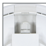
dławnica zapewniająca IP66
