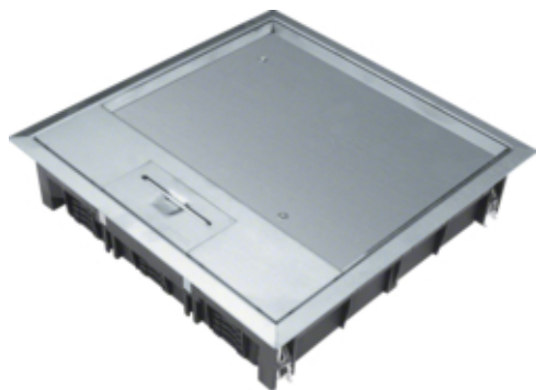
tehalit.VE-EE Pokrywa uchylna VEQ12 244x244 wykładzina 12mm stal nierdzewna
