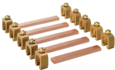
univers Łącznik szyn zbiorczych 12x5mm 5-pol. 40mm
