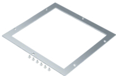
tehalit.UK Pokrywa montażowa dla UD roz.2 Q12 244x244mm stal ocynkowana
