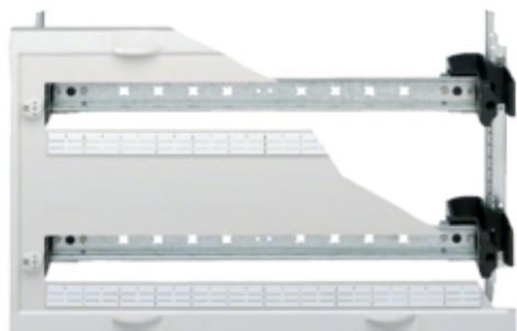
univers N Blok dla aparatów modułowych montowanych poziomo 2x24M 300x500mm
