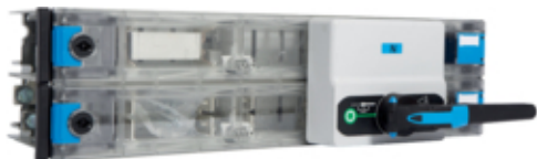
LLD-1 rozł. izol. z bezp. 3P+N 250A 400VAC odp.lewy AC22B
