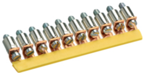
Mostek równoległy 10-polowy do zacisków 6mm 2
