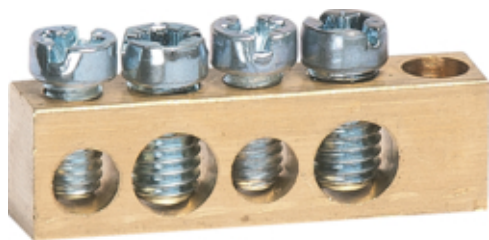
Listwa przyłączeniowa bez wspornika 2x16 + 2x10 mm 2
