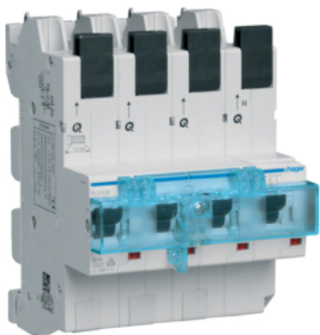
MCB SLS Wyłącznik nadprądowy selektywny 3P+N, Cs, 16 A, szyny Cu 40-12x5/10mm
