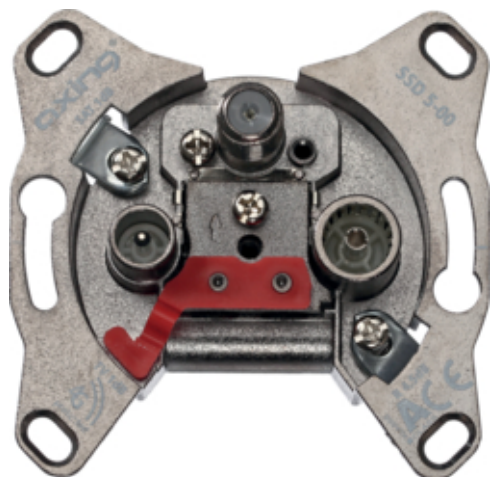
tehalit.WA Mechanizm gniazda RTV-SAT przelotowego 10dB 5-2200MHz
