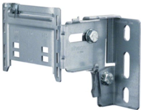
tehalit.BR/BRN Odstępnik uniwersalny odległość od ściany 53-81mm
