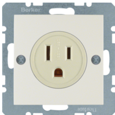
B.Kwadrat/S.1 Gniazdo z uz. USA/KANADA NEMA 5-15 R, krem
