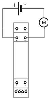
Bezpośredni pomiar wartości obwodów prądu stałego.
