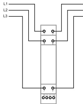
Bezpośredni pomiar natężenia prądu sieci trójfazowej.
